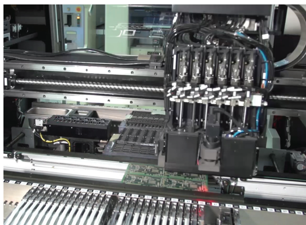
Osazování čipů
